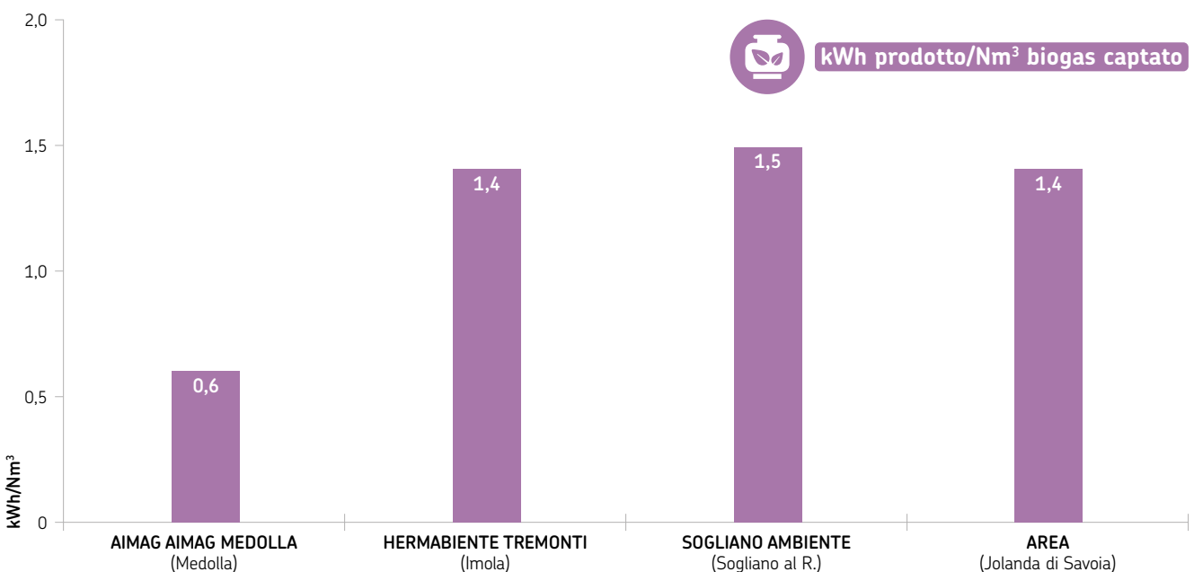
FIGURA 7 Energia prodotta (kWh) per Nm 3 di biogas captato nelle discariche operative, anno 2024
