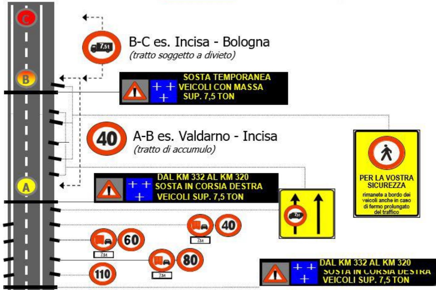
schema planimetrico
