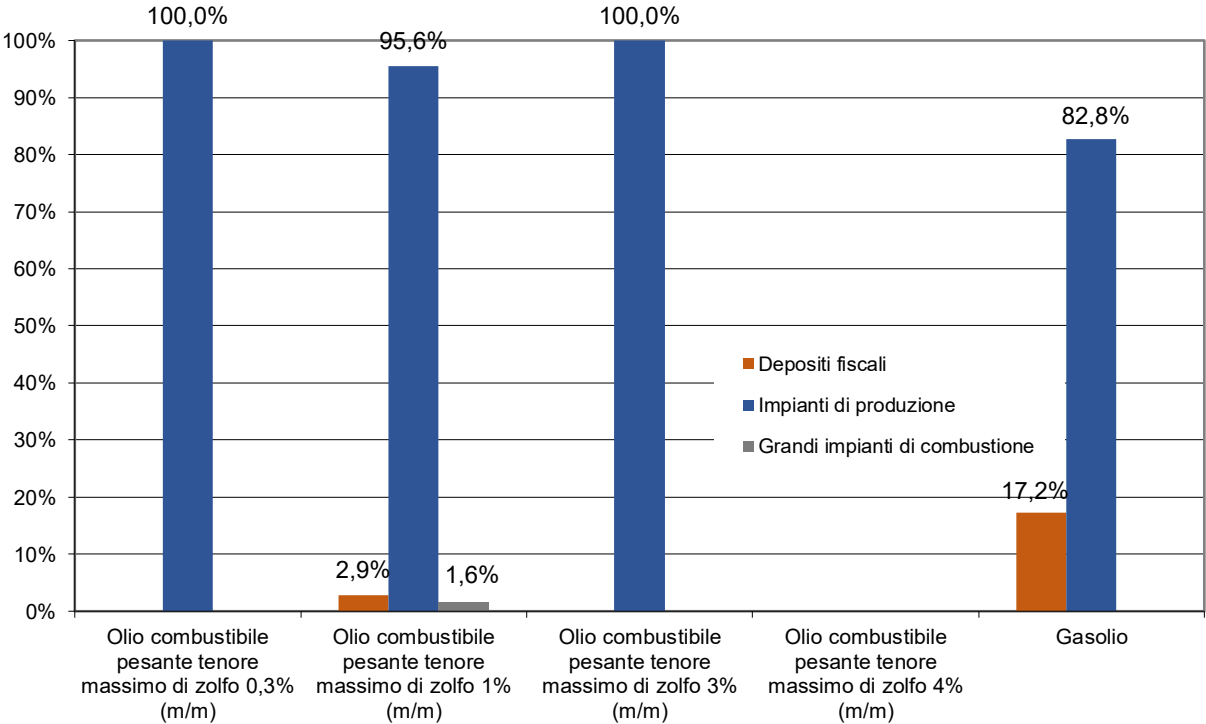
Fig.4.4 Olio combustibile pesante e gasolio prodotti e importati nel 2024, con l'esclusione dei quantitativi destinati all'esportazione e l'inclusione dei quantitativi utilizzati all'interno dell'impianto. Ripartizione percentuale in funzione del tipo di olio e del tipo di impianto
