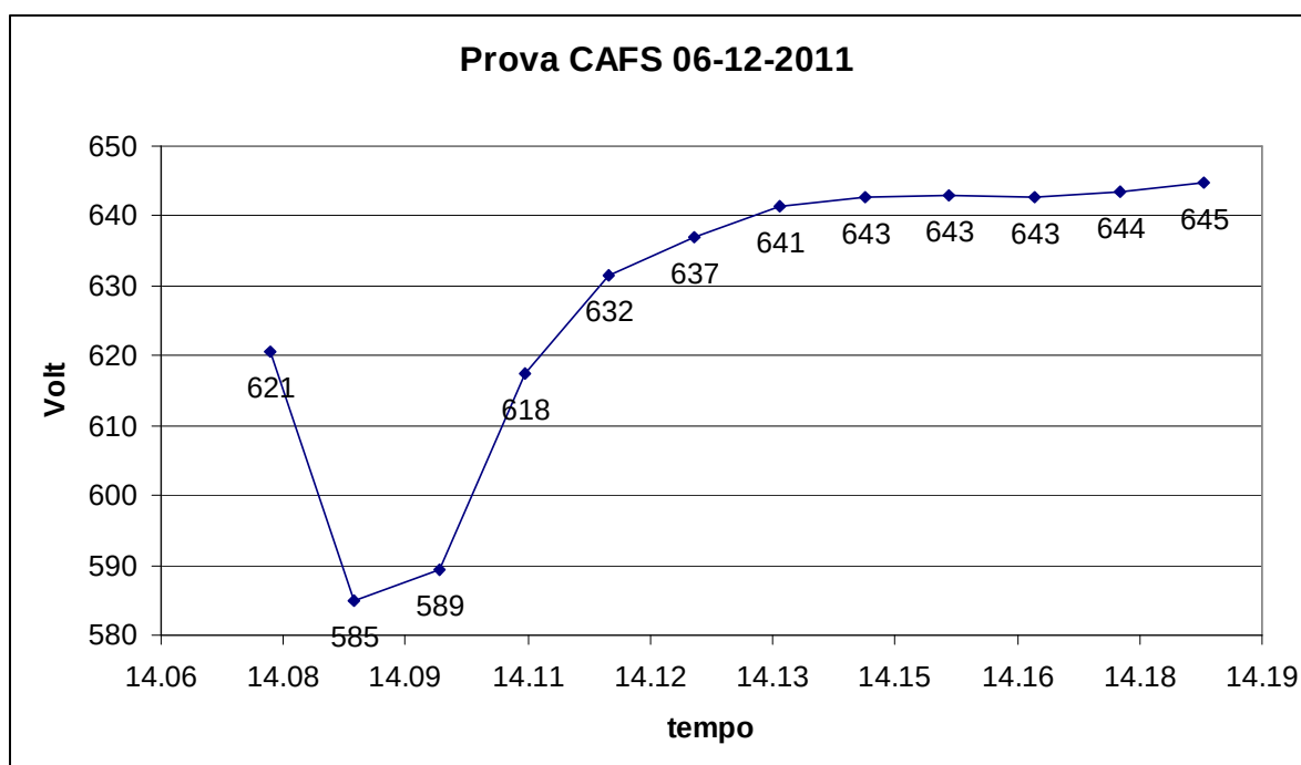
Figura 5-8: grafico con l'andamento delle tensioni
