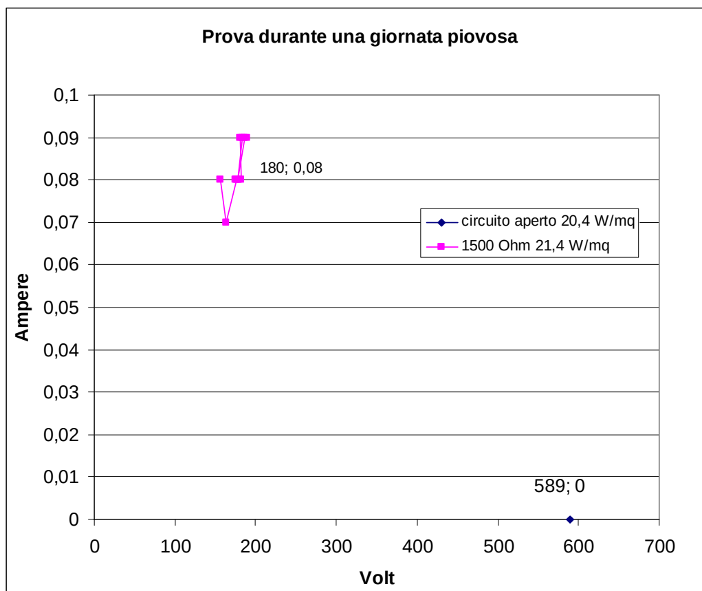
Figura 5-38: Grafico delle tensioni e correnti durante una giornata piovosa
