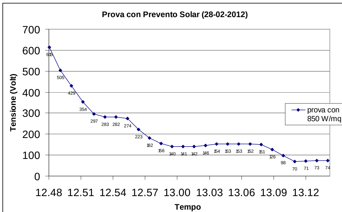
Figura 5-28: prova con Prevento Solar
