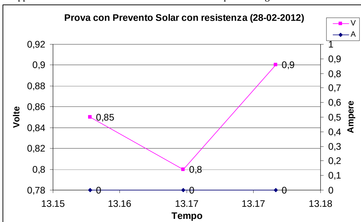
Figura 5-29: prova con Prevento Solar: valori di tensione e corrente con i pannelli coperti
