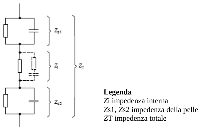
Figura 3-1: rappresentazione dell'impedenza interna del corpo umano
