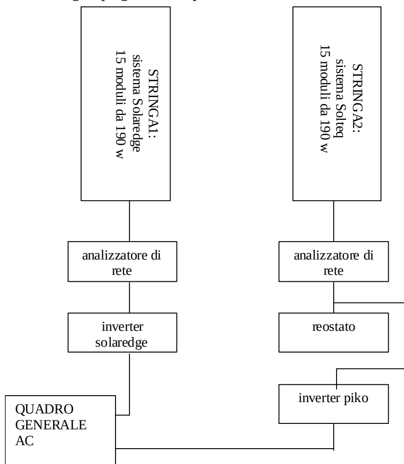
Figura 4-3: schema a blocchi del funzionamento dell'impianto fotovoltaico sperimentale.
