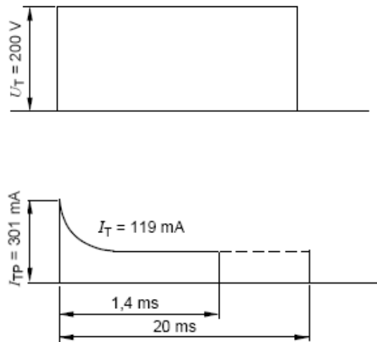
Figura 3-4: Oscillogramma della tensione di contatto U_T e della corrente I_T in corrente continua, percorso di corrente da mano a mano, superficie di contatto estesa, in condizioni asciutte
