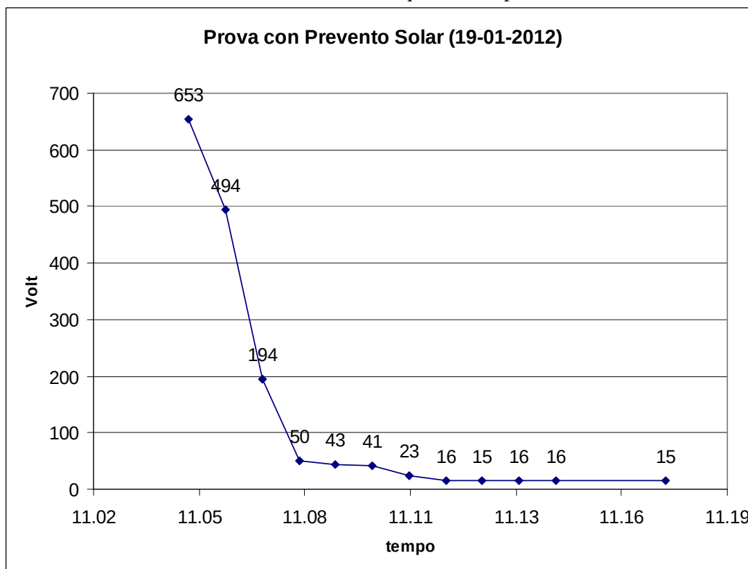
Figura 5-20: prova con PreventoSolar
