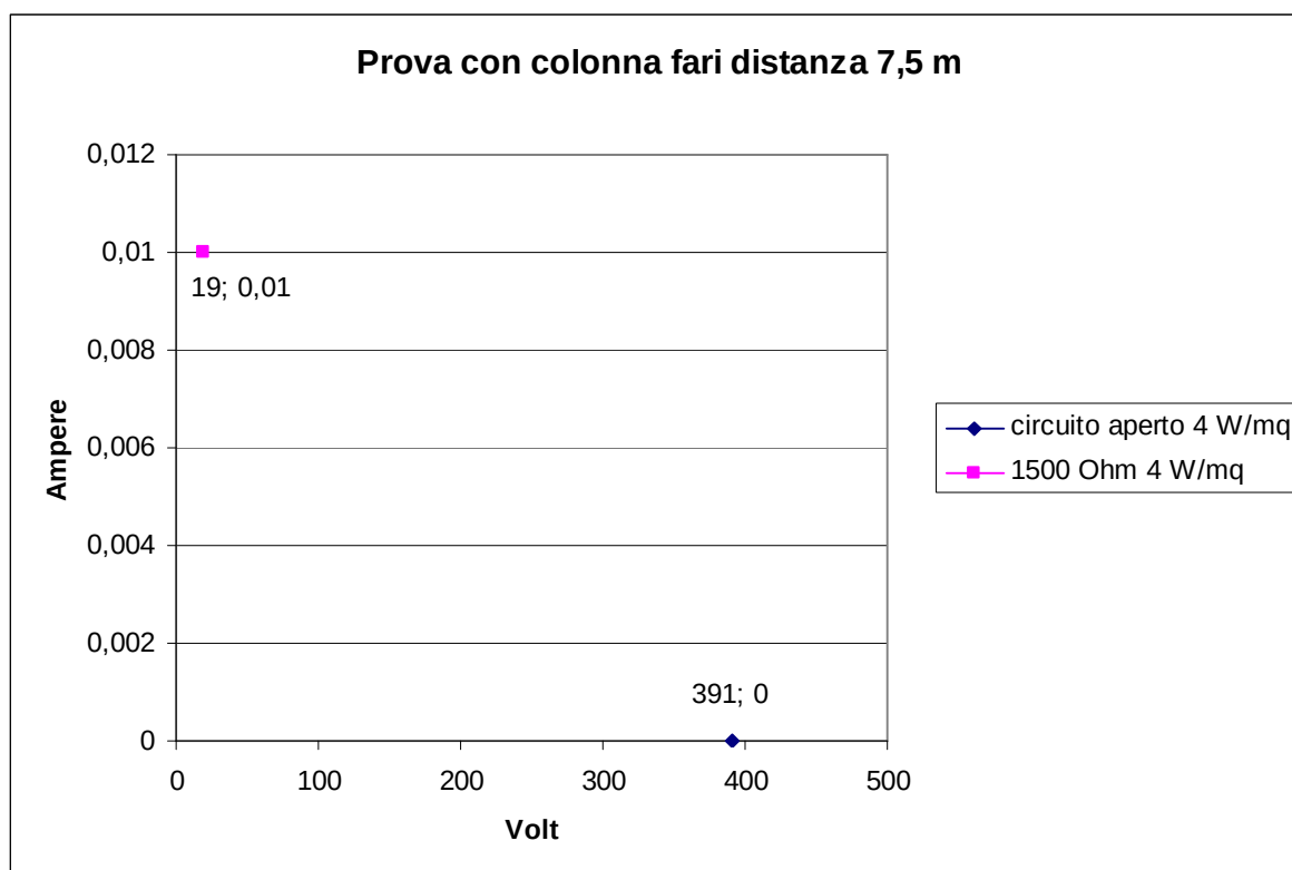
Figura 5-40: prima prova: colonna fari distante 7,5 m dalla stringa in prova
