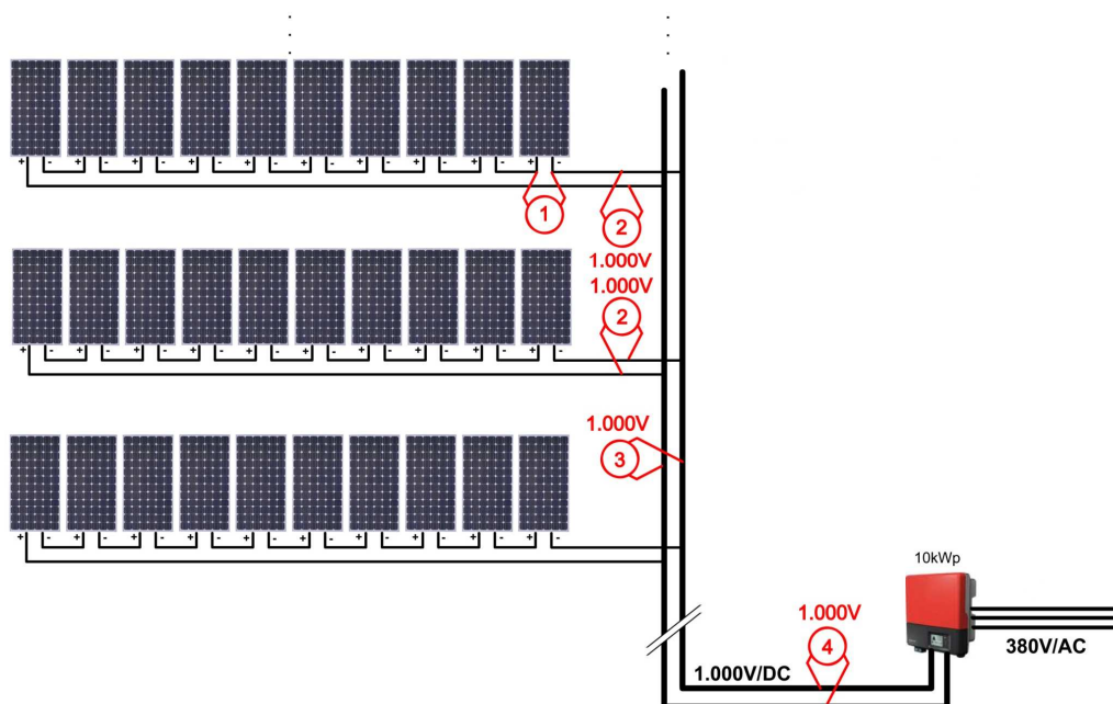
Figura 2-2: schema di un impianto fotovoltaico
