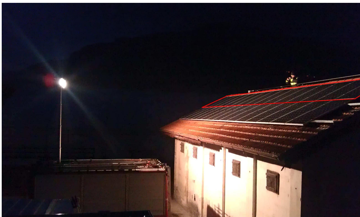
Figura 5-39: prima prova: colonna fari distante 7,5 m dalla stringa in prova
