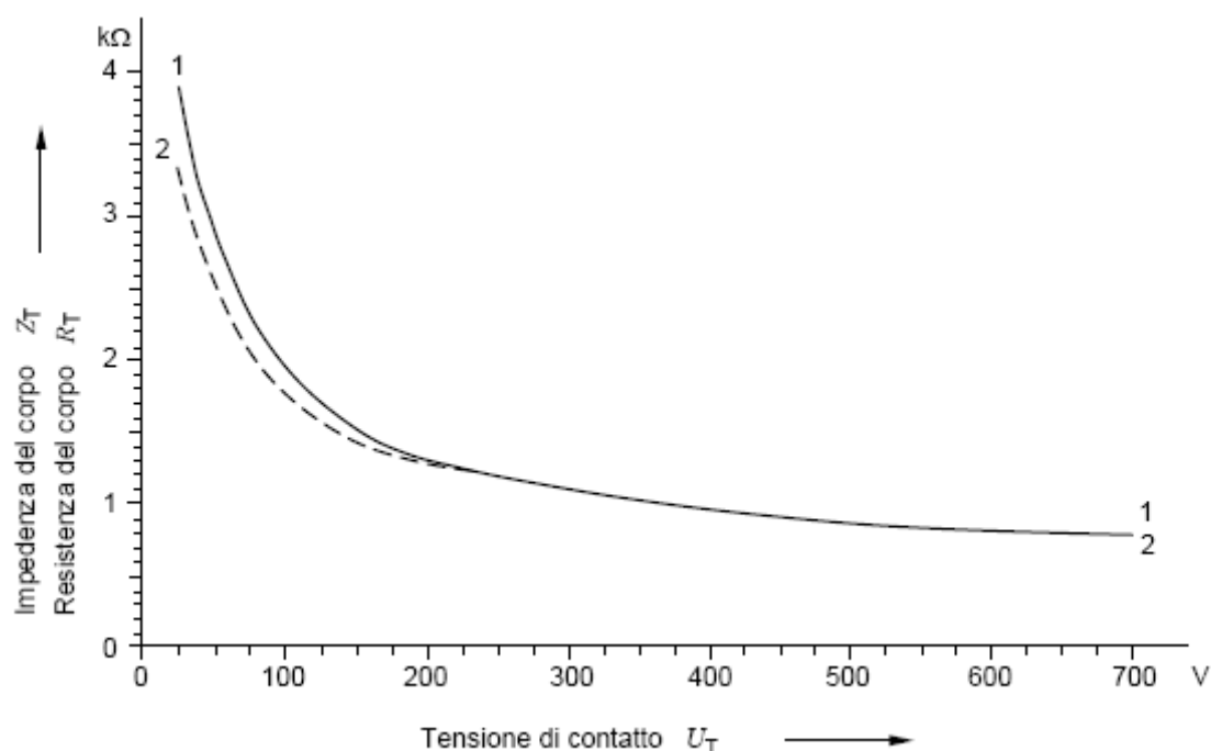
Figura 3-8: Valore statistico delle impedenze totali del corpo Z_T (corrente alternata a 50 Hz) e della resistenza del corpo R_T (corrente continua) per una percentuale del 50 % di una popolazione di esseri umani viventi, in un percorso di corrente da mano a mano, con aree della superficie di contatto estese, in condizioni di asciutto, per tensioni di contatto sino a 700 V, in corrente alternata a 50/60 Hz (2) e in corrente continua (1)
