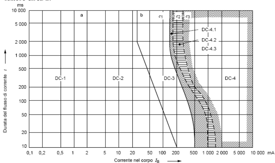
Figura 3-5: Zone tempo/corrente convenzionali degli effetti delle correnti continue su persone, per un percorso di corrente longitudinale ascendente
