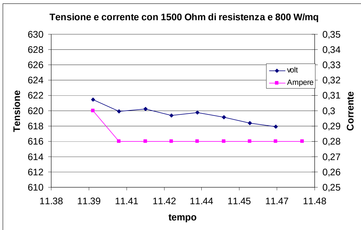
Figura 5-2: prova in condizioni standard con 1500 Ohm di resistenza
