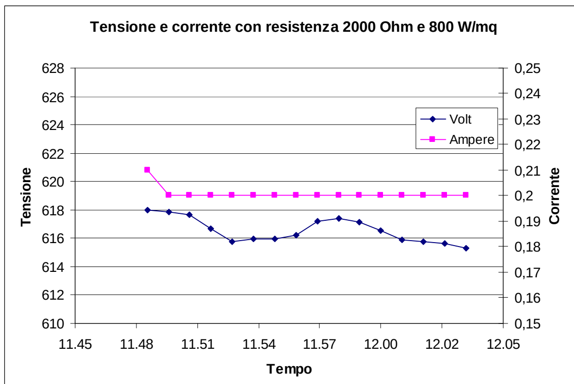
Figura 5-1: prova in condizioni standard con 2000 Ohm di resistenza
