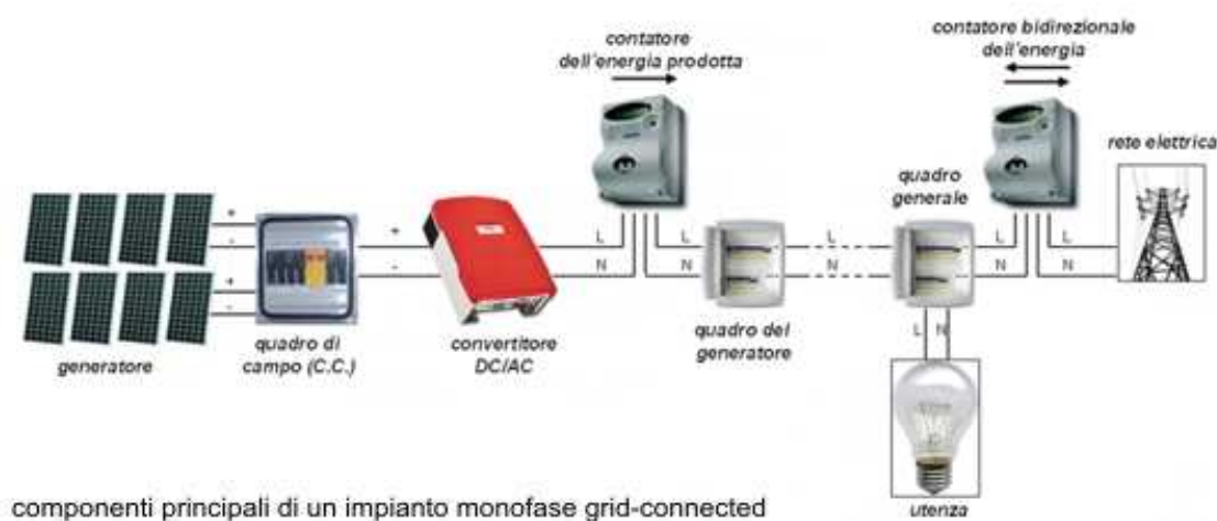
Figura 2-1: schema di un impianto fotovoltaico
