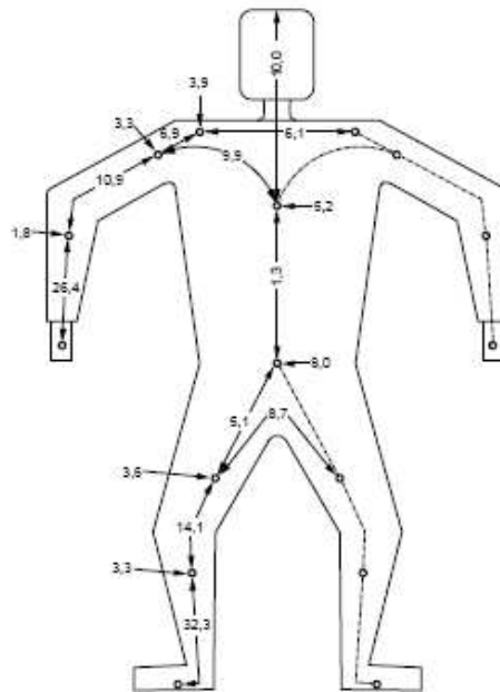
Figura 3-2: percentuale d'impedenza interna
