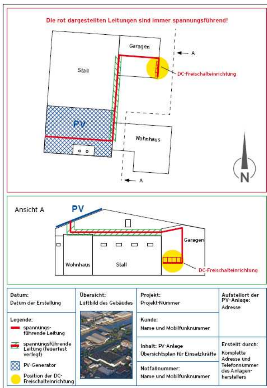
Figura 1-2: schema dell'impianto fotovoltaico
