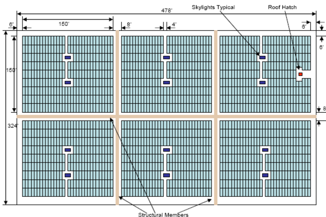
Figura 1-5: esempio posizionamento dei pannelli fotovoltaici
