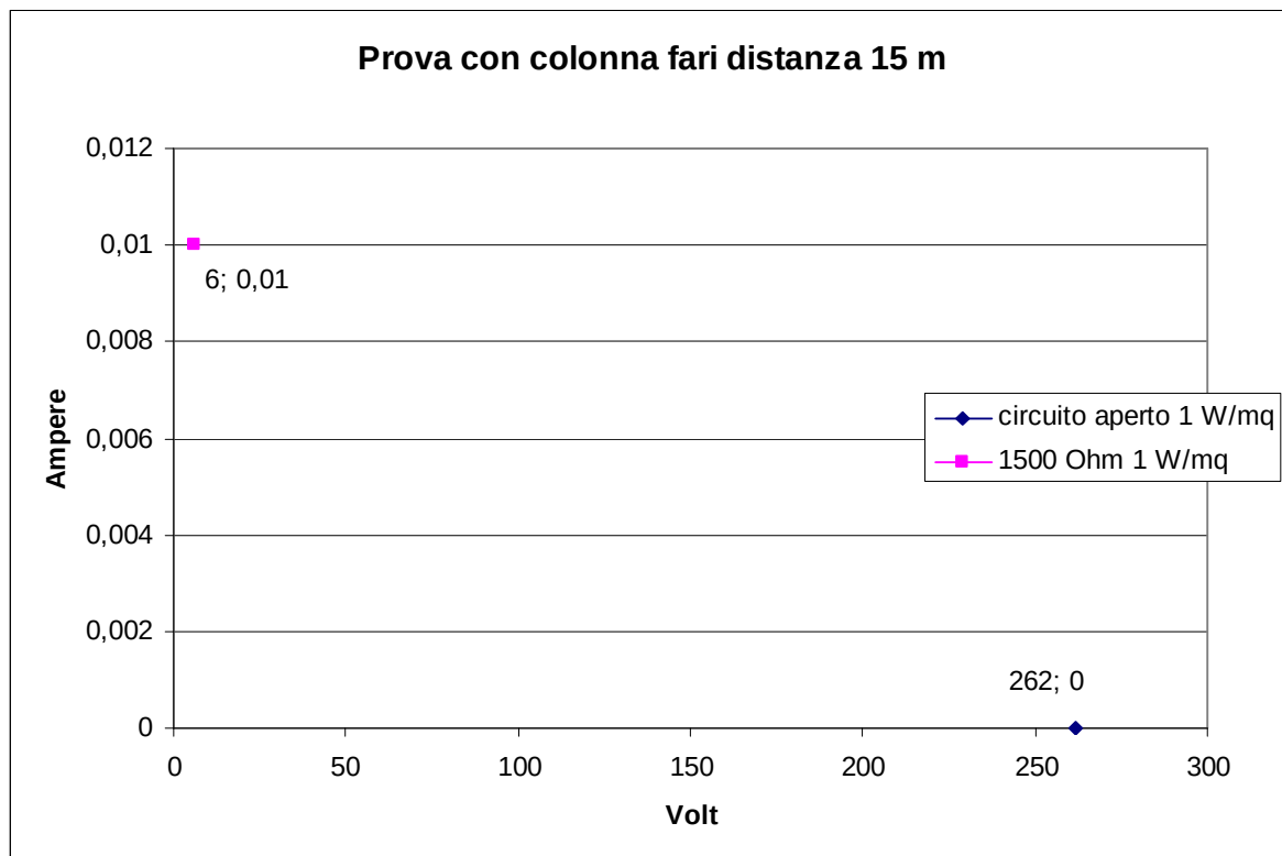
Figura 5-45: seconda prova: colonna fari distante 15 m dalla stringa in prova
