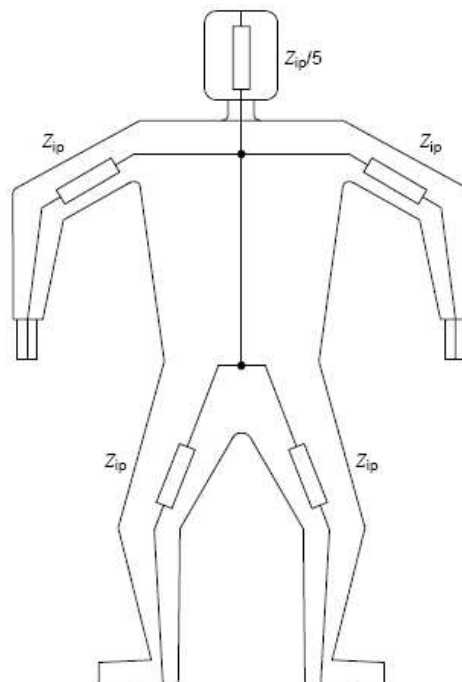
Figura 3-3: Schema semplificato delle impedenze interne del corpo umano
