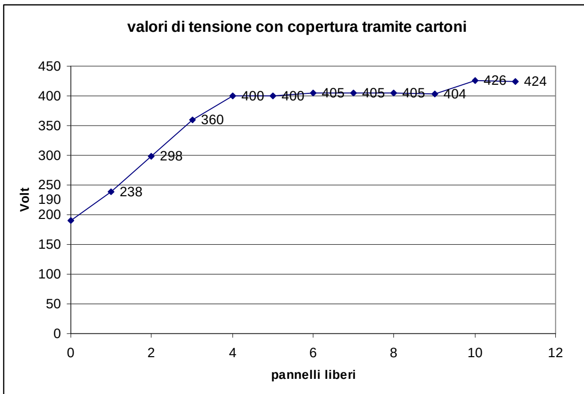
Figura 5-9: grafico con l'andamento delle tensioni
