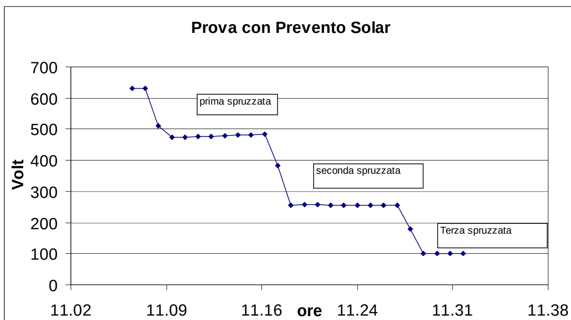
Figura 5-13: prova con PreventoSolar
