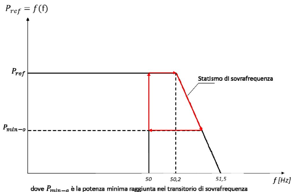
Figura 11 – Curva di sola riduzione della potenza attiva in sovrافrequenza
