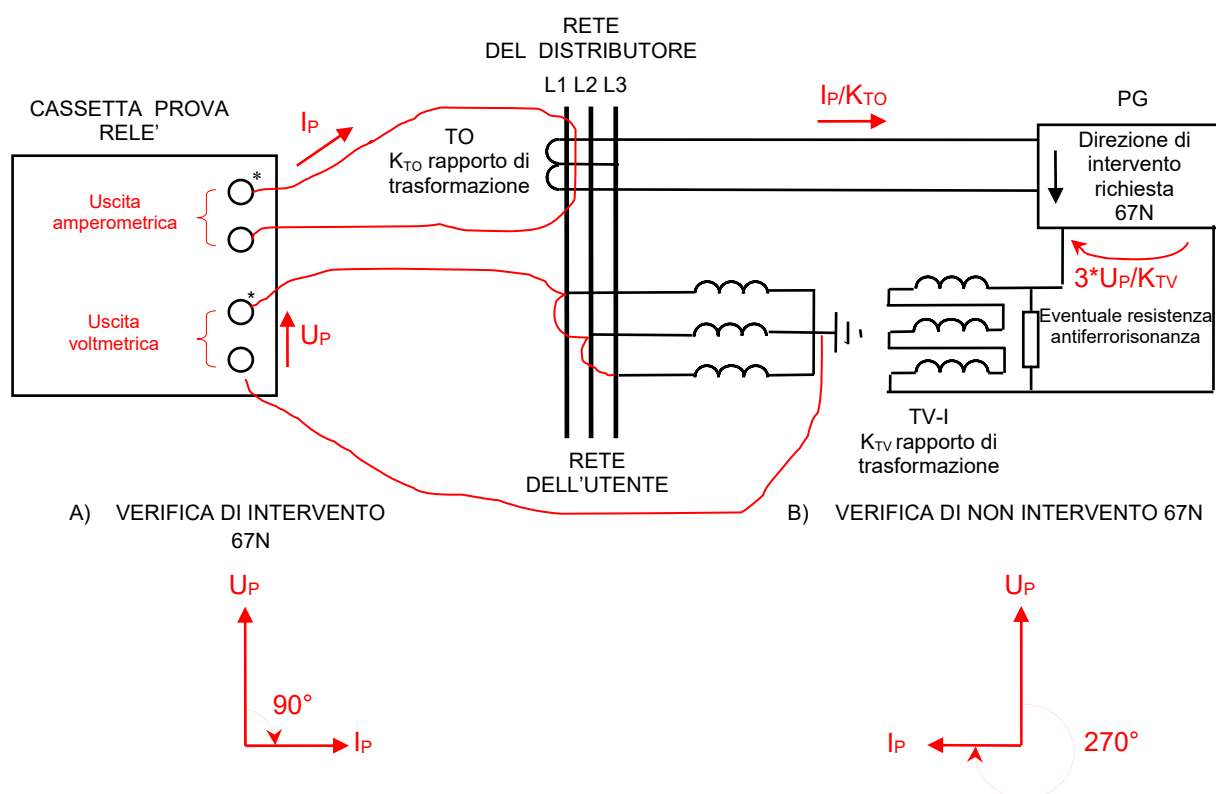
FIGURA 2.bis: schema di principio per la verifica di direzionalità della protezione 67N. Lo schema si riferisce ad un SPG con misura di corrente residua mediante TO sommatore e misura di tensione residua mediante TV-I stella-triangolo aperto. Per SPG che misura la tensione residua come somma vettoriale delle tre tensioni di fase misurate mediante TV-I o TV-NI, le connessioni voltmetriche della cassetta prova relè al primario dei TV-I o TV-NI sono identiche a quelle in figura. Per SPG che misura la corrente residua come somma vettoriale delle tre correnti di fase misurate mediante tre TA-NI amperometrici, le connessioni amperometriche della cassetta prova relè sono identiche a quelle in figura con la sola eccezione che l'iniezione deve avvenire al primario di uno solo dei tre TA-NI.
