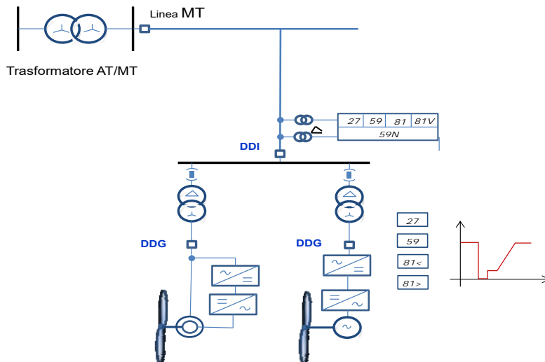
Figura 35 – Protezione dei generatori eolici Tabella 33
