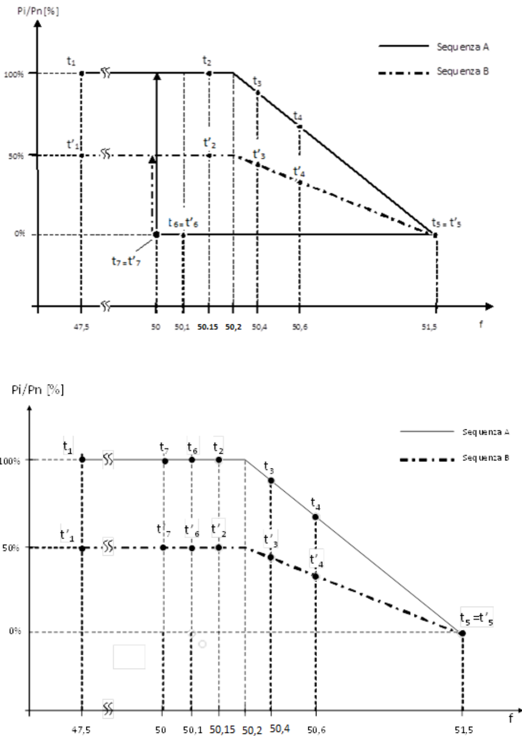
Figura 22 – Curve di limitazione della potenza attiva rispetto alla frequenza per generatori statici (in alto) e per i generatori eolici (in basso)
