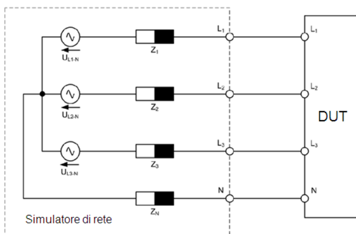
Figura 28 – Utilizzo di simulatore di rete
