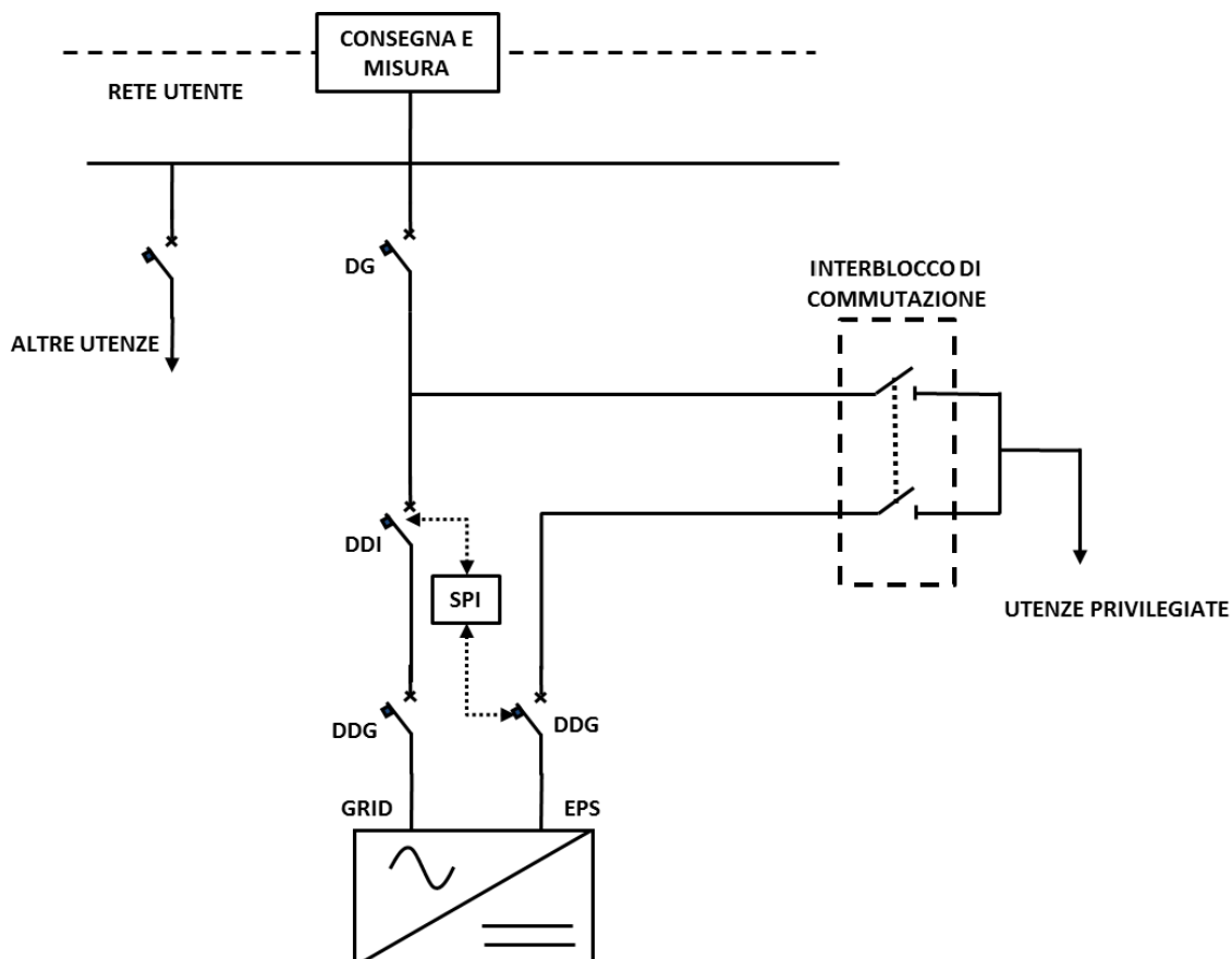
Figura 11a – Esempio di sistema di produzione di energia con funzionamento in isola attraverso porta dedicata
