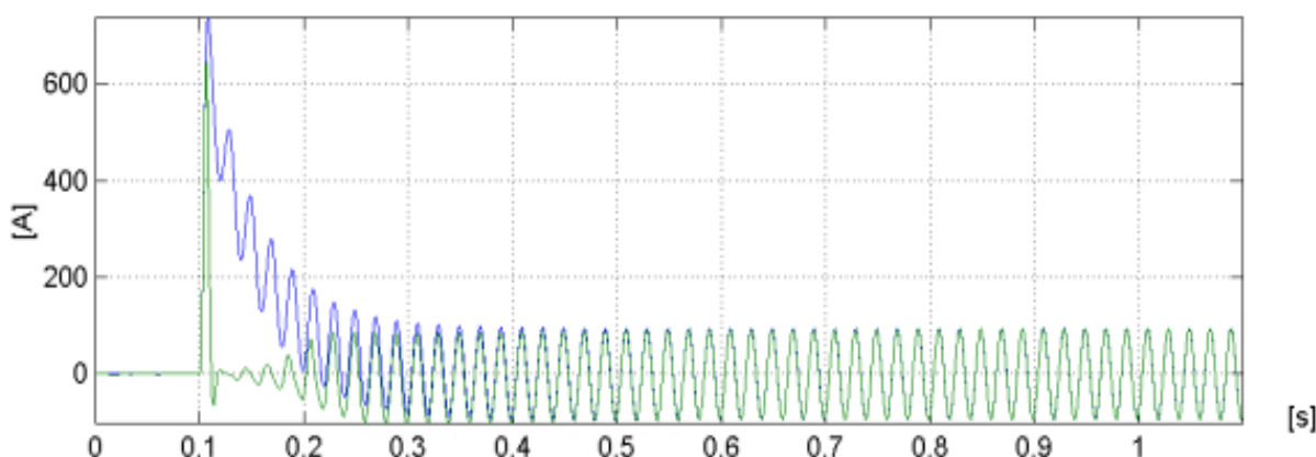
Figura 2 – Corrente secondaria convenzionale per TA omopolari (TO)
