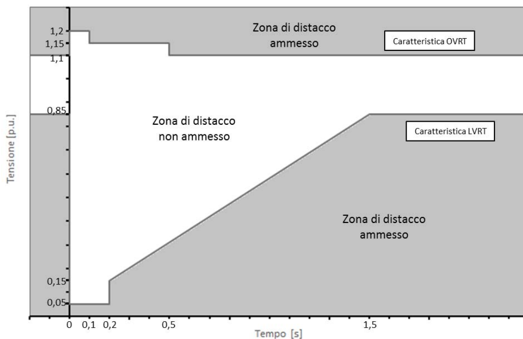
Figura 25 – Caratteristica (V - t): LVRT e OVRT per generatori eolici
