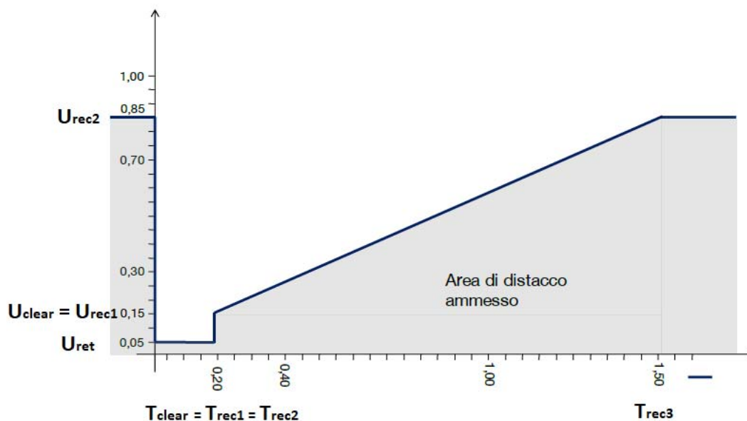
Figura 19b – Profilo di fault-ride-through dei parchi di generazione
