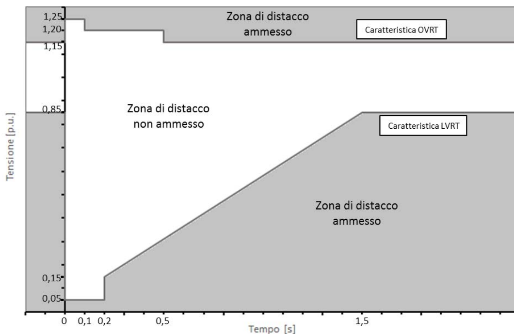
Figura 20a – Caratteristica (V - t): LVRT e OVRT per i generatori statici
