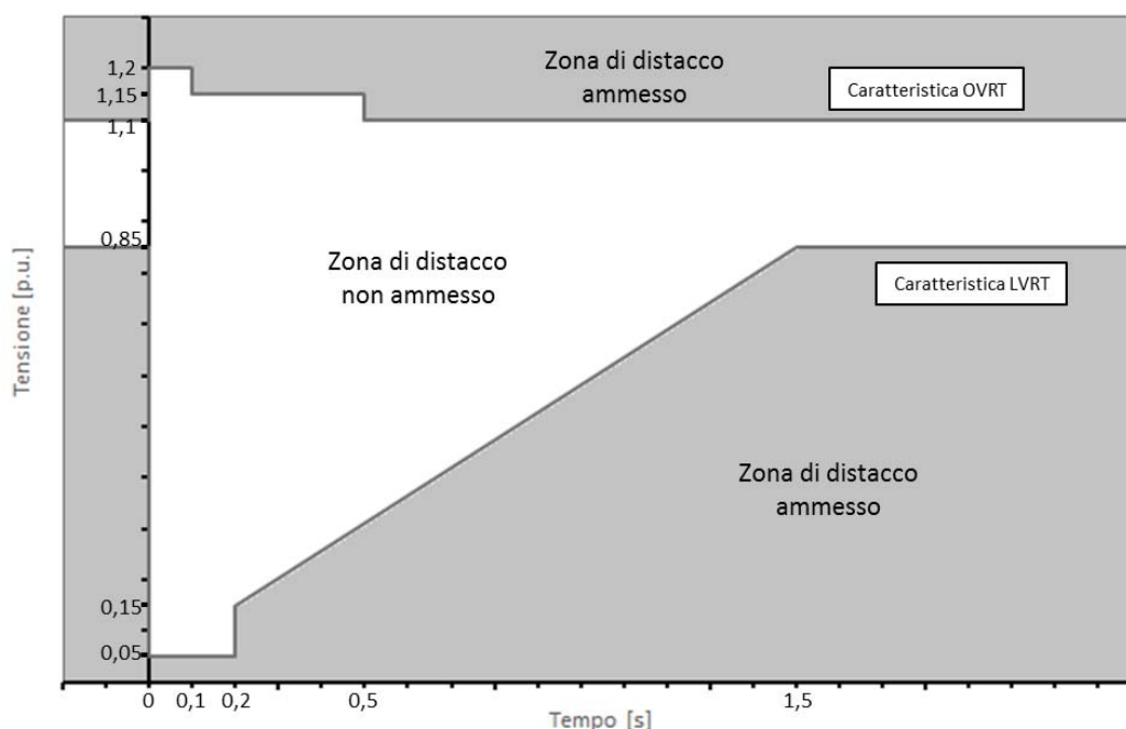
Figura 20b – Caratteristica (V - t): LVRT e OVRT per generatori eolici.
