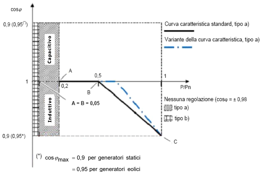
Figura 9 – Curva caratteristica standard \cos\phi = f(P) e varianti, definite su tre punti
