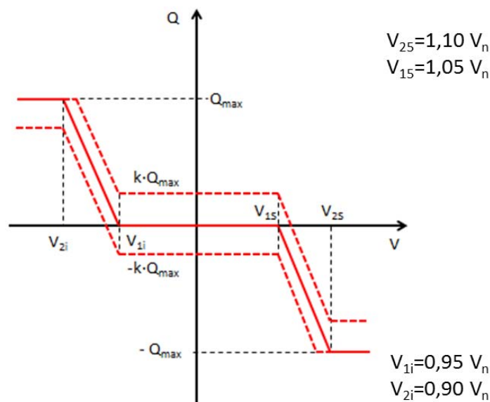
Figura 31: Curva caratteristica Q = f(V) .
