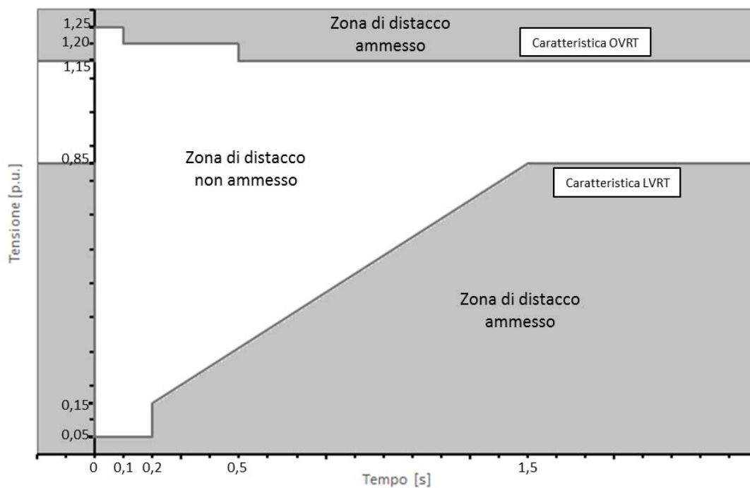
Figura 8 – Caratteristica (V - t): LVRT e OVRT
