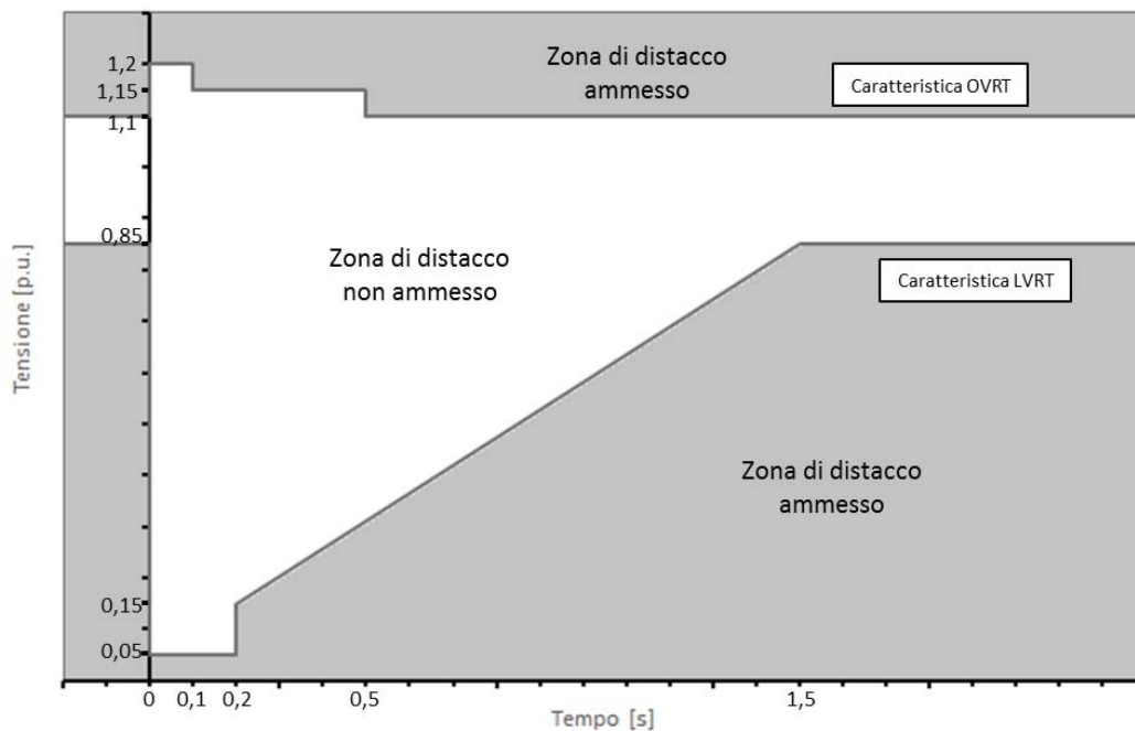
Figura 36 – Caratteristica FRT dei generatori eolici
