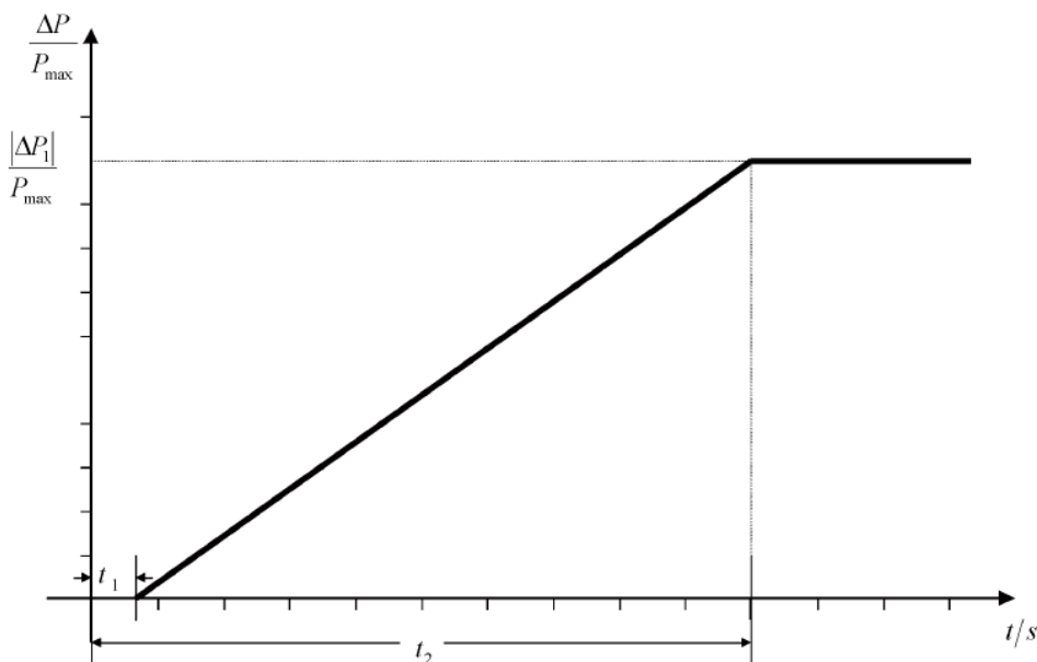
Figura 29: Capacità di risposta frequenza/potenza attiva. Pmax è la potenza massima alla quale si riferisce ΔP
