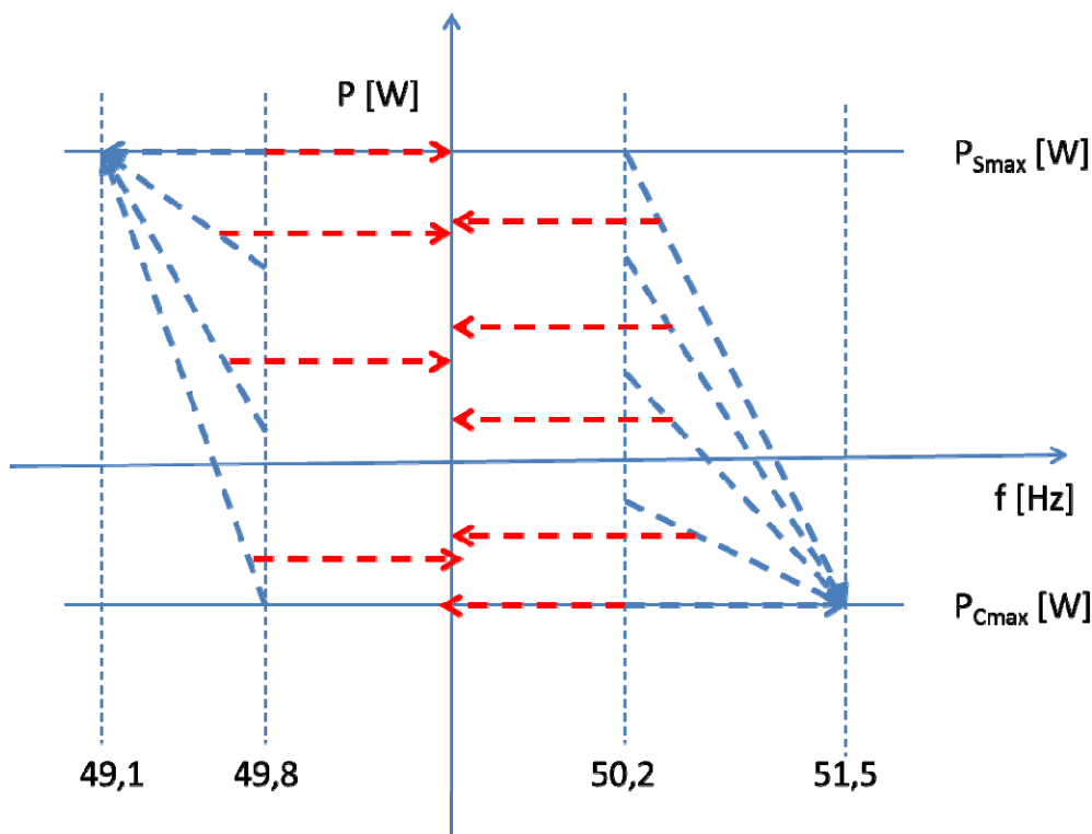
Figura 21-b – Rientro da condizioni di sovra e sottofrequenza
