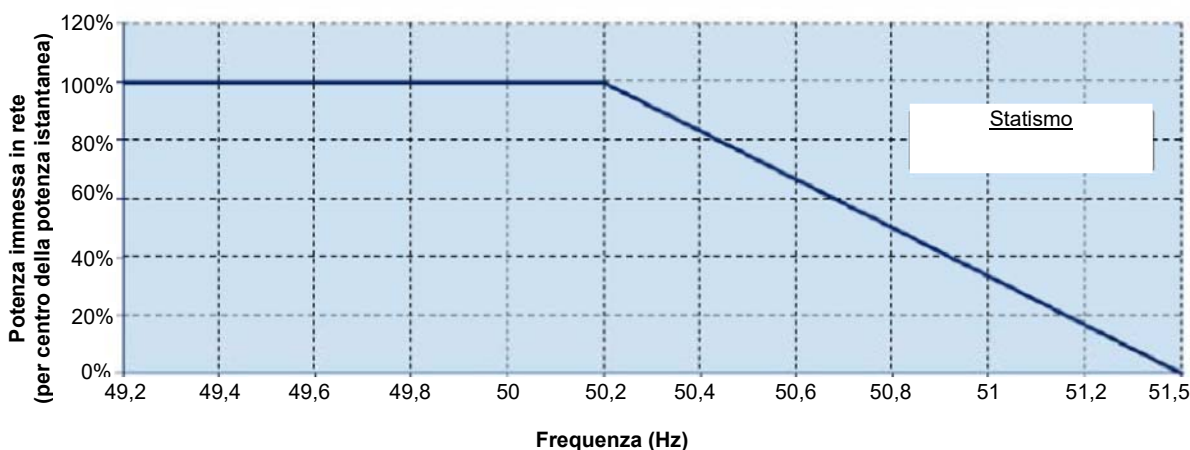
Figura 21 – Regolazione della potenza attiva immessa in rete in condizioni di sovralfrequenza
